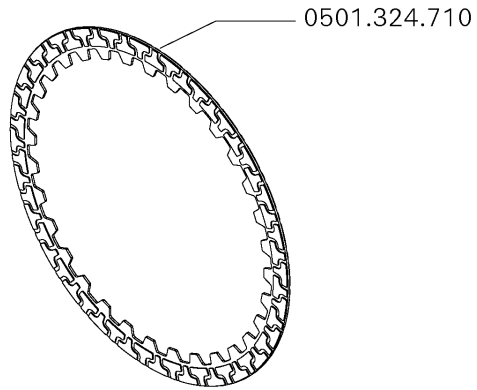
Bremse A
