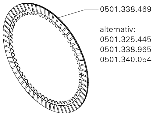
Kupplung D
